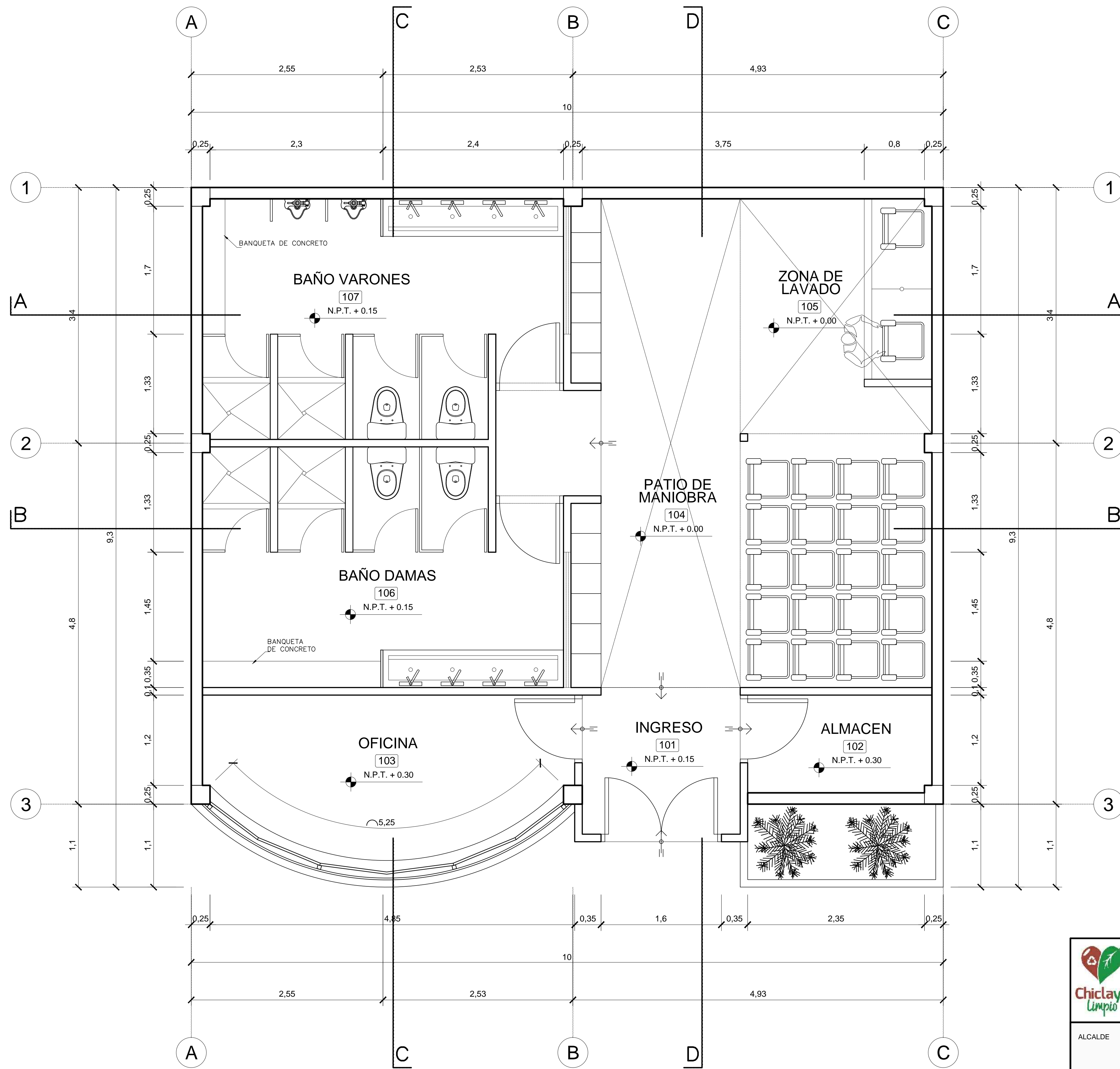
PLANTA DISTRIBUCION ESC:1/50
